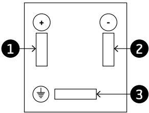
Power Electrical DIN Connector [Controller]
