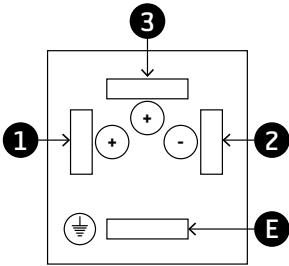
Power Electrical DIN Connector [Terminal Strip]
